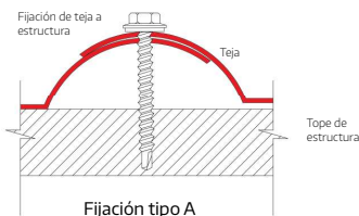
Fijación tipo A
