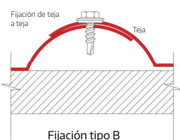
Fijación tipo B
